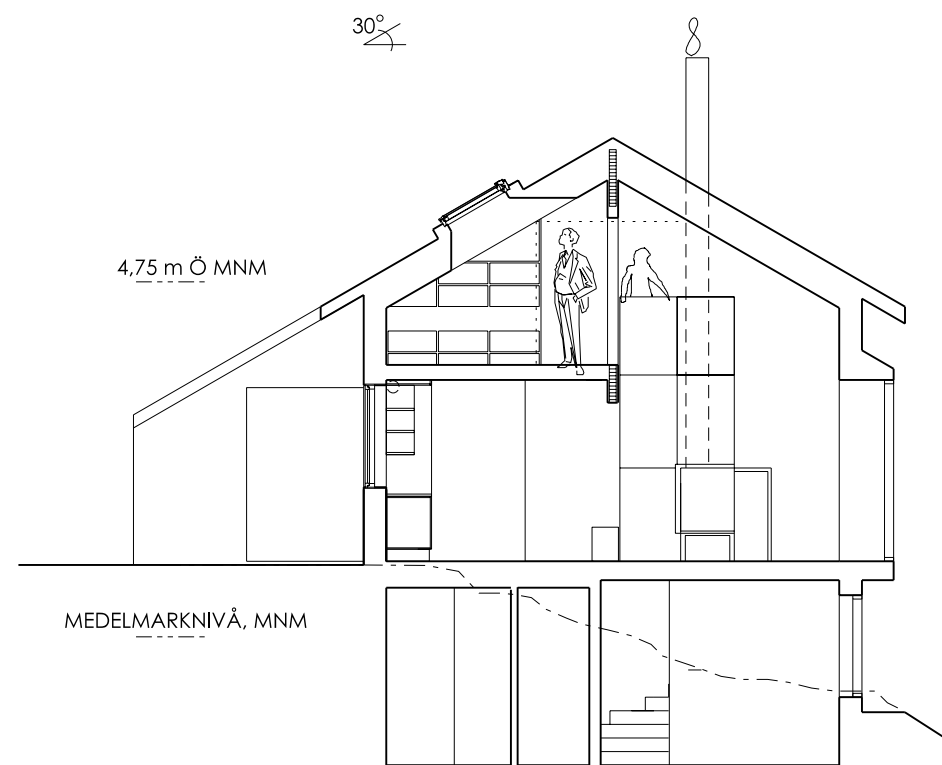
SEKTION C-C
