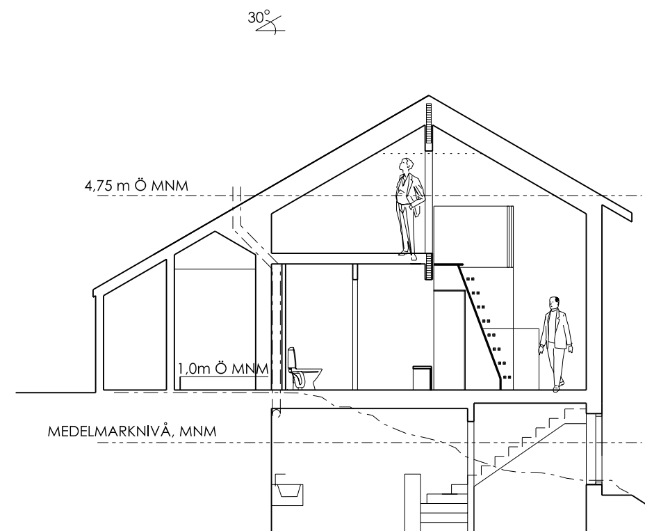
SEKTION B-B
